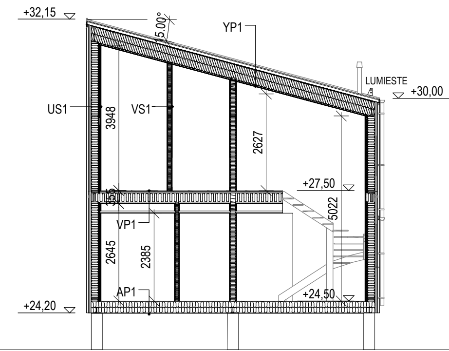
Leikkaus
